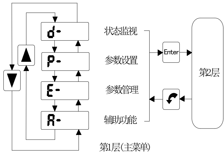
图 4-2 第一层菜单方式选择操作框图
