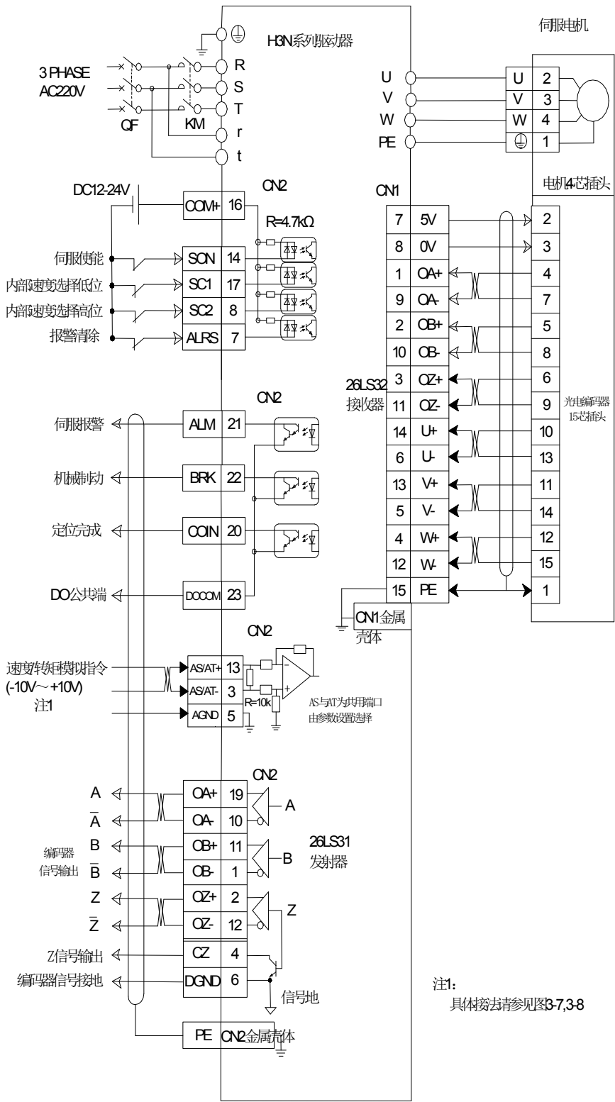
图 3-14 速度/转矩模拟量控制下标准接线图
