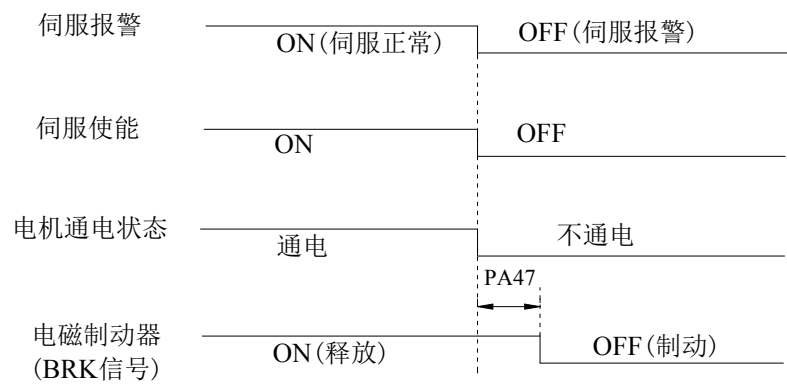
图 5-12 伺服驱动器静止状态下报警时序图
