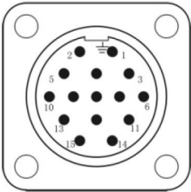
电机航空插头示意图
