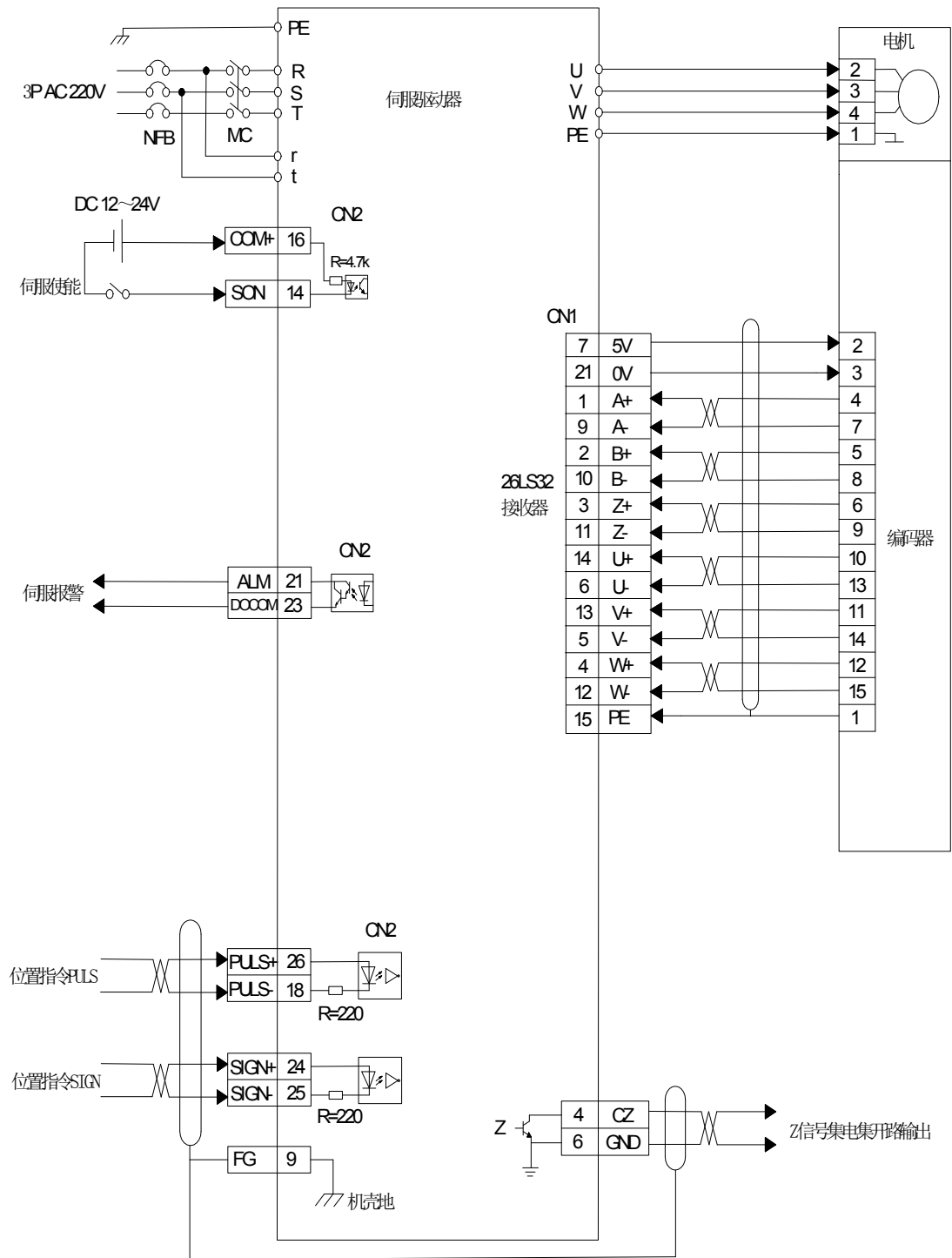
图 5-3 简单位置定位系统接线图
