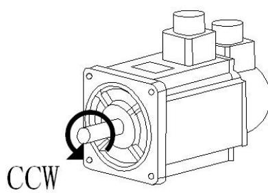
图 2-3 伺服电机旋转方向定义
