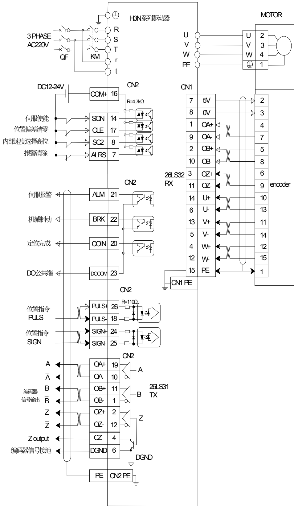
图 3-13 位置控制下标准接线图
