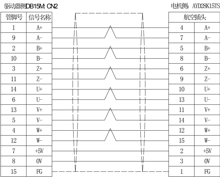
ROLLON 系列驱动器与电机编码器连接
