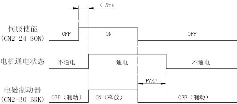
图 5-10 伺服驱动器静止使能时序图
