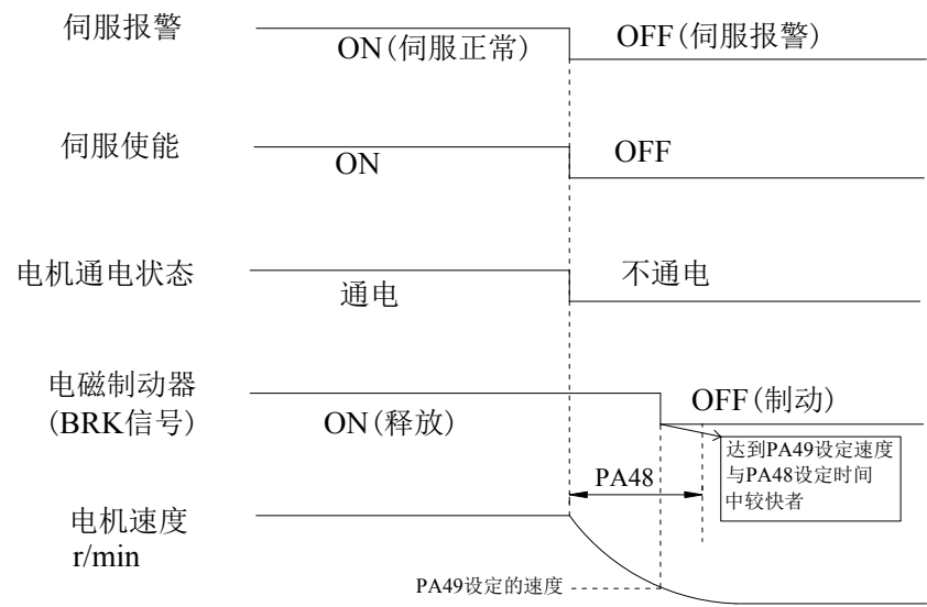
图 5-13 伺服驱动器运动状态下报警时序图
